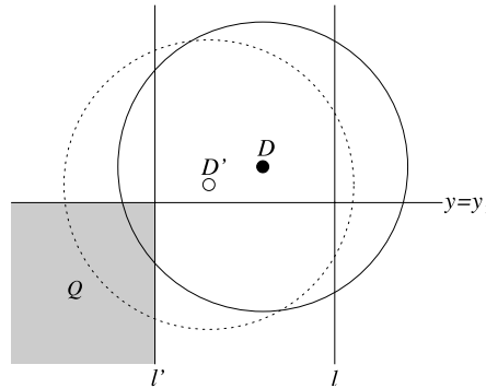
Fig. 2. If D dominates D' at l and D' dominates D at l' , then D \cap Q \subseteq D' \cap Q .
